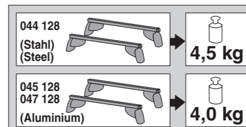
Art.-Nr. / Part-No. : 044 128 (Stahl / Steel)
